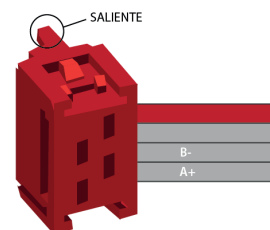
Figura 10 Conector RS-485
