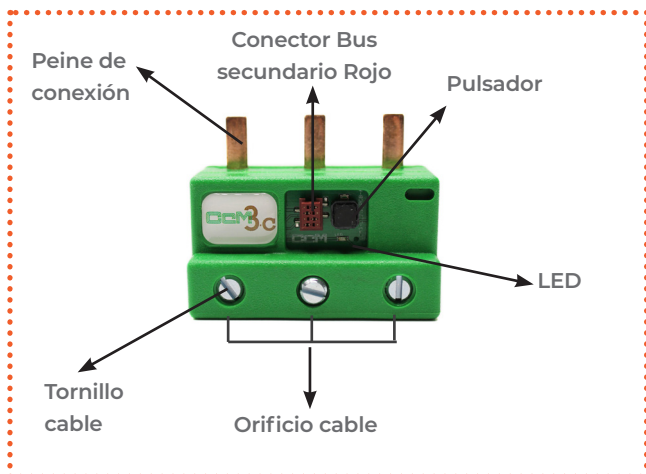
Figura 2 Descripción gráfica CEM3-C .
