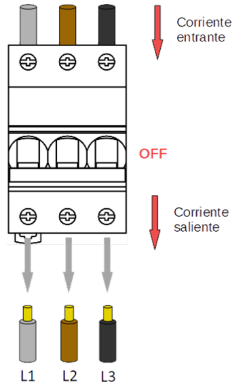
Figura 6 Desconexión de las líneas de corriente
